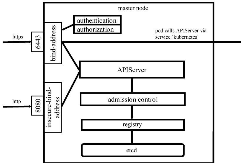
图8-3 一个正在运行的APIServer的拓扑结构
