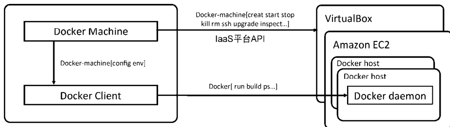
图6-3 Machine工作流程
