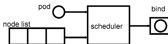
图8-4 把调度器看成一个黑盒
