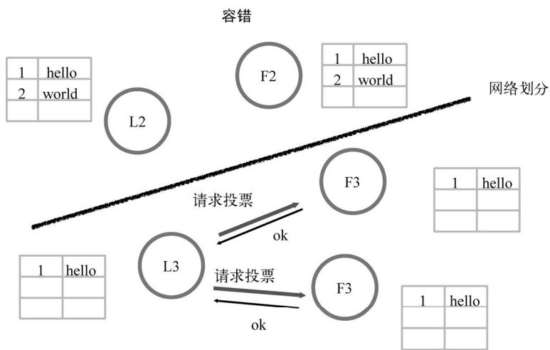
图4-28 节点宕机
