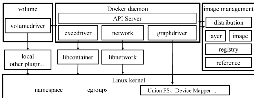
图3-8 Docker架构总览
