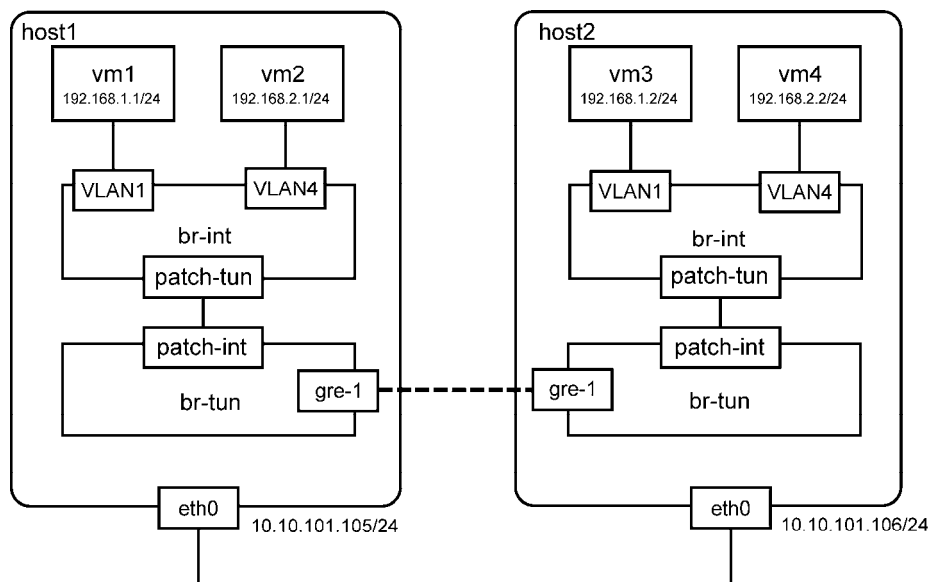
图4-15 OpenStack的GRE网络模型
