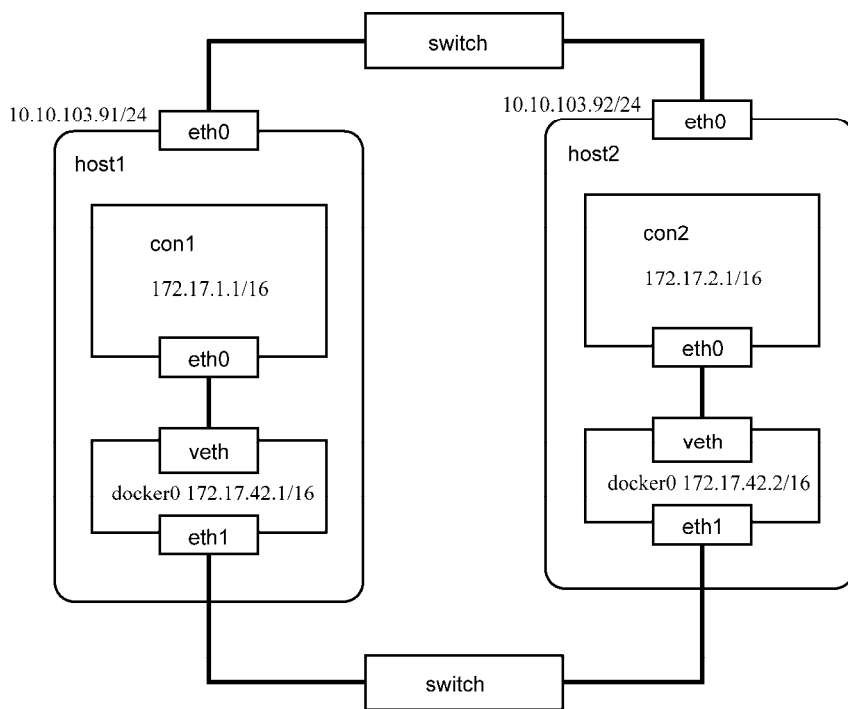
图4-3 桥接网络拓扑图
