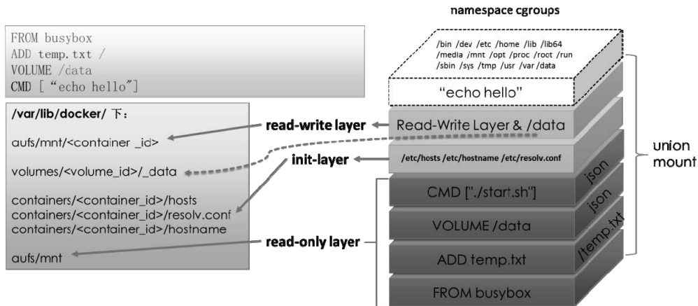
图3-12 Docker容器文件系统的全局视图
