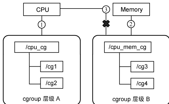
图3-5 一个已经附加在某个层级上的子系统不能附加到其他含有别的子系统的层级上
