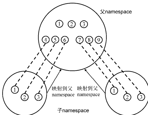
图3-3 namespace映射图 ①
