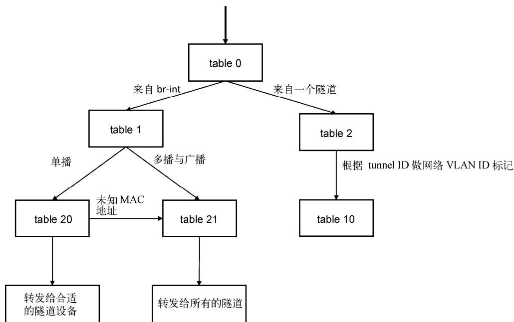
图4-16 br-tun网桥流表匹配流程
