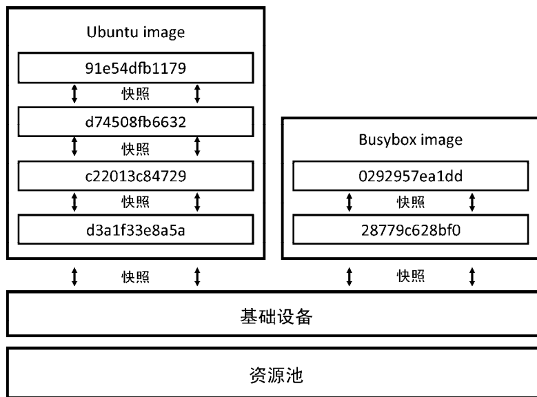
图3-15 devicemapper镜像层结构示意图 ①
