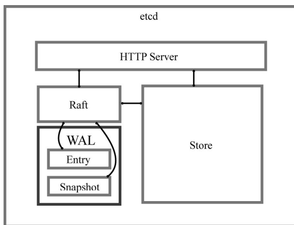
图4-24 etcd架构图
