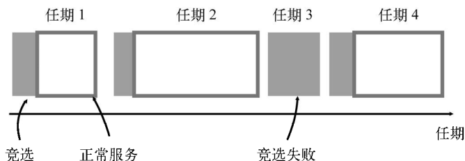
图4-26 任期示意图
