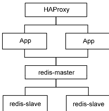
图2-2 Docker应用栈结构图
